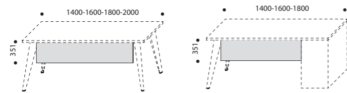
L. 1400/1600/1800/2000
