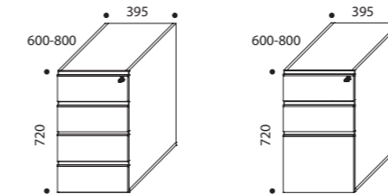
L. 395 D/P. 600/800
