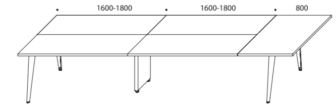
L. 4000/4400 D/P. 1600
