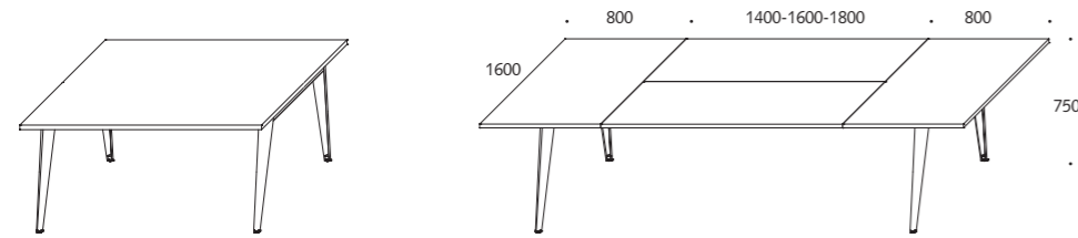
L. 1600 D/P. 1600
