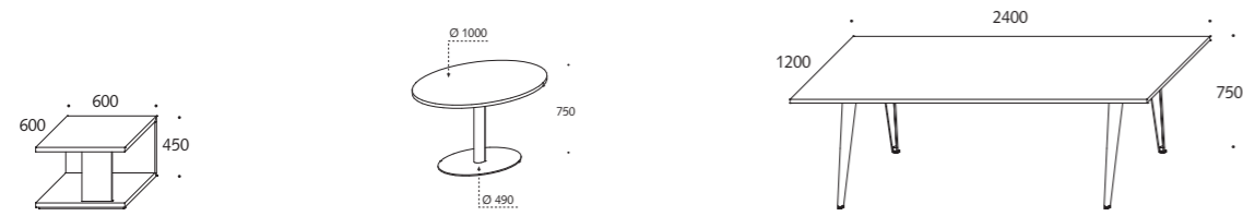
L. 600 D/P. 600
